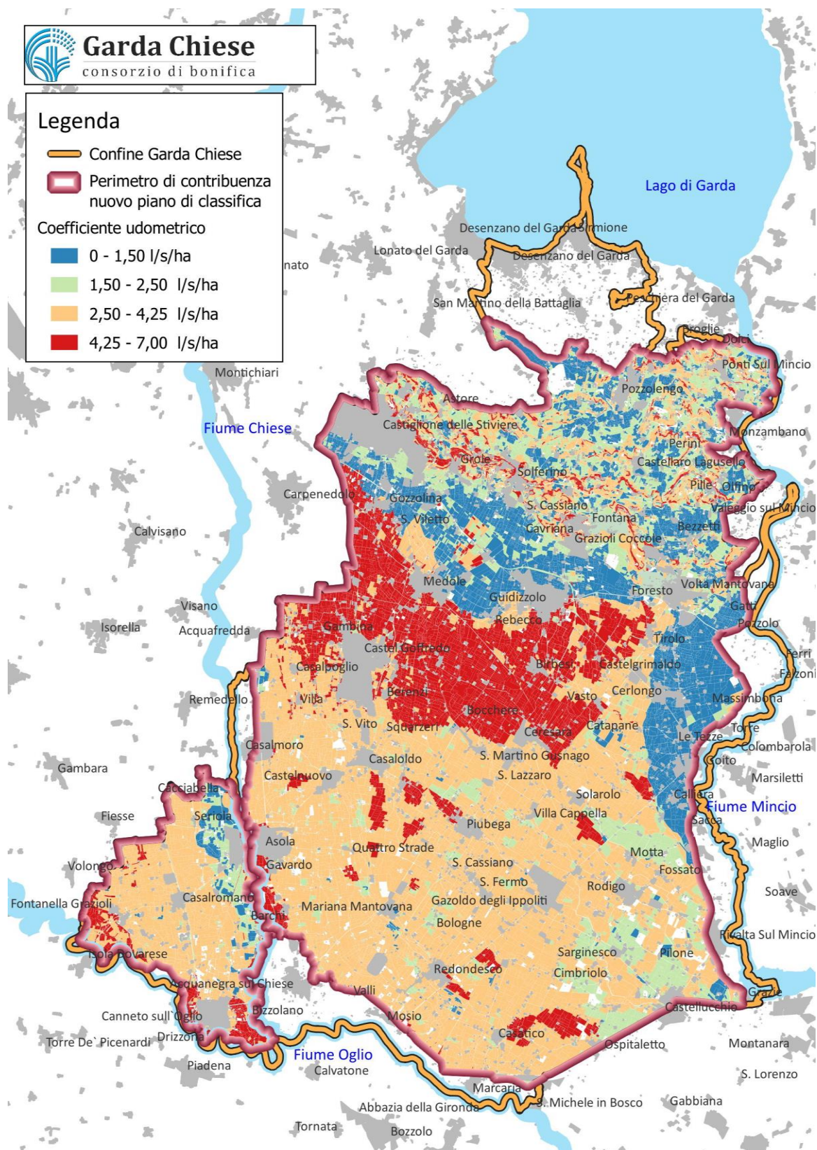
Fig. 3.11 – Suddivisione dei terreni secondo 4 classi omogenee di produzione di deflusso
