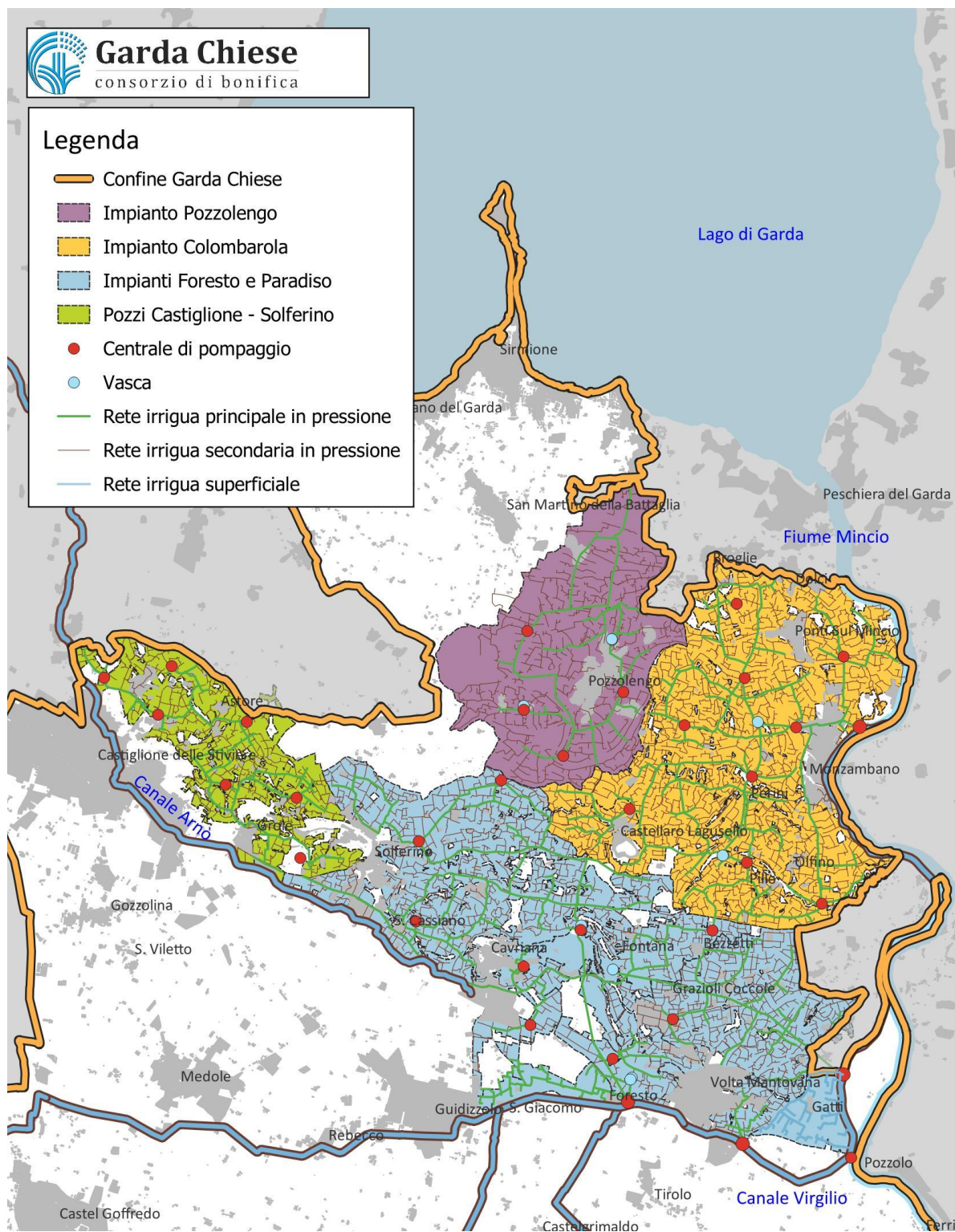
Fig. 4.7 – Sottobacini irrigui della zona dei Colli Morenici
