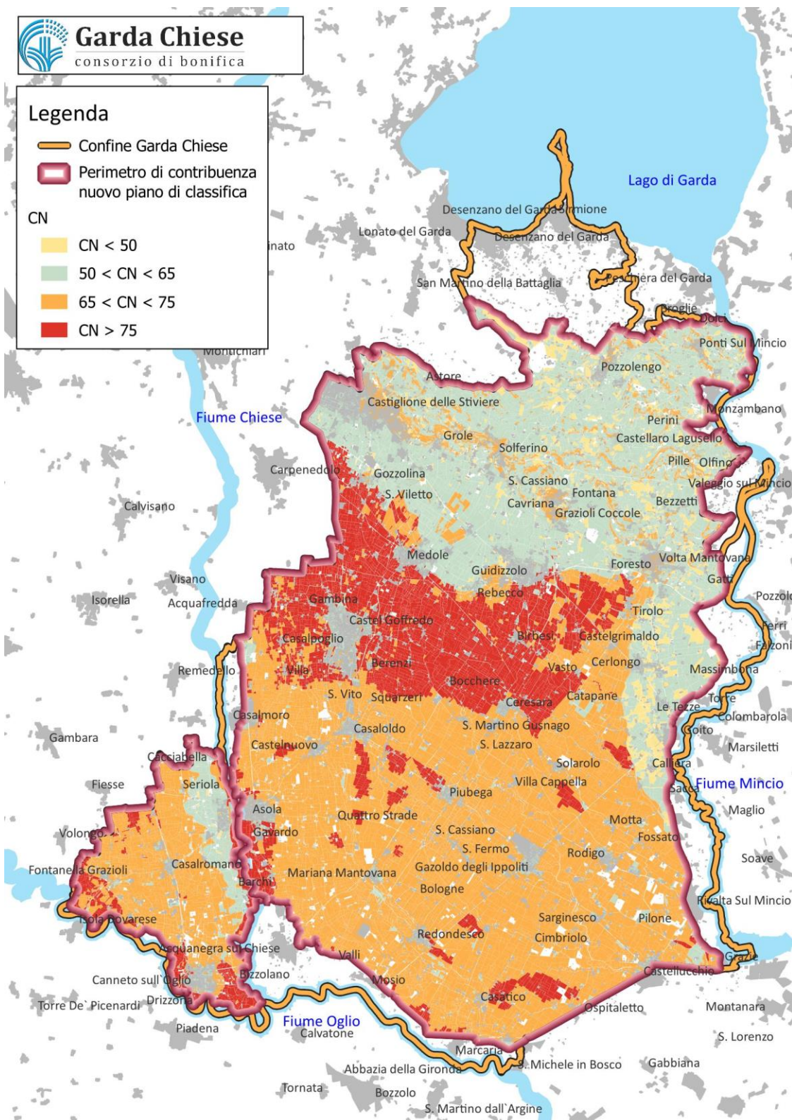
Fig. 3.10 – Planimetria dei CN
